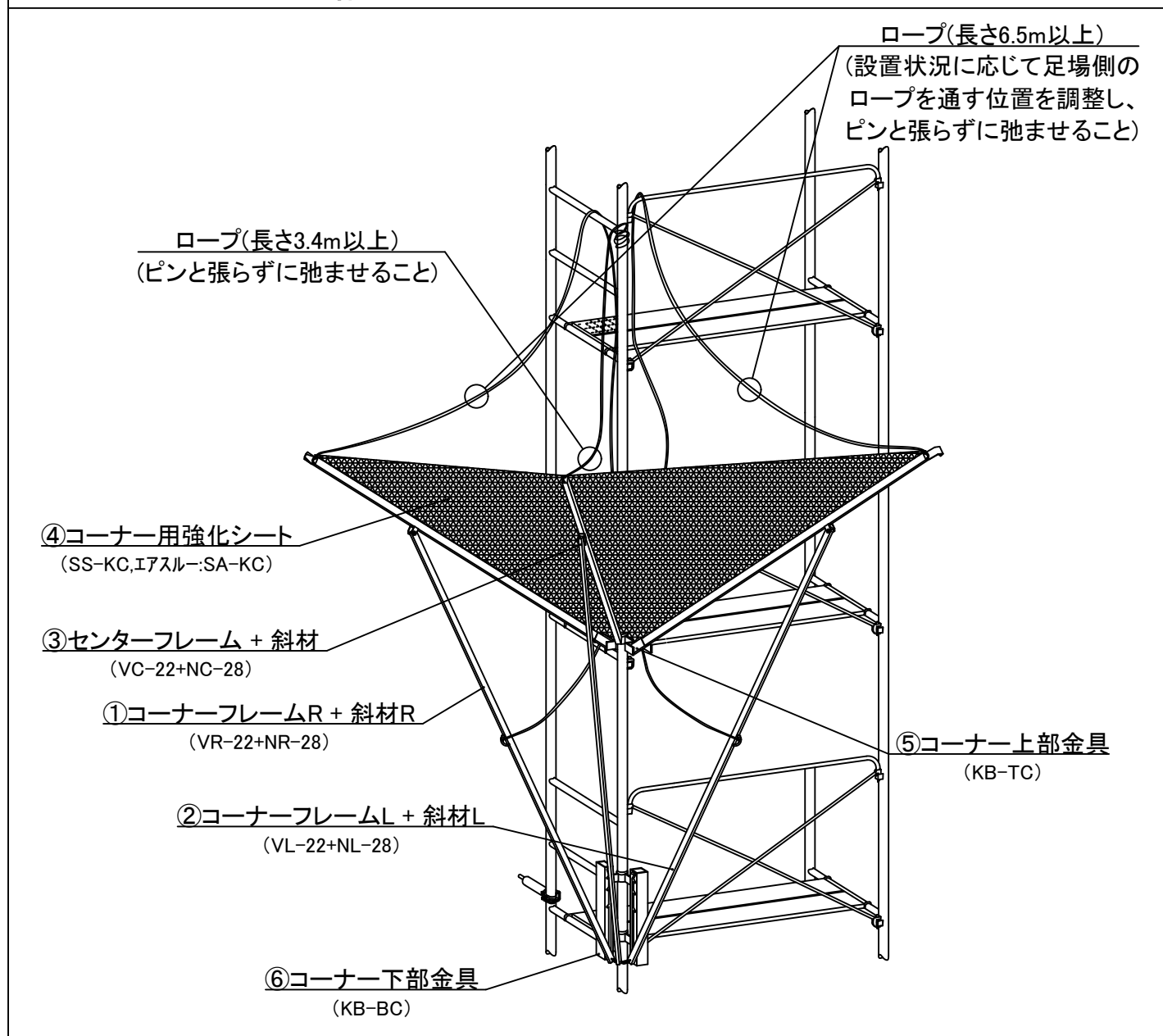
構成部材図（コーナー部）
