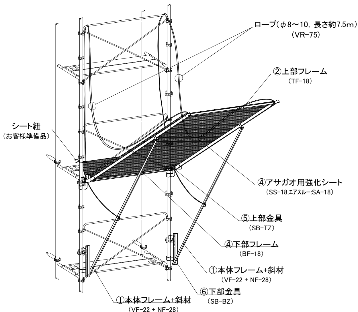
構成部材図（直線部）
