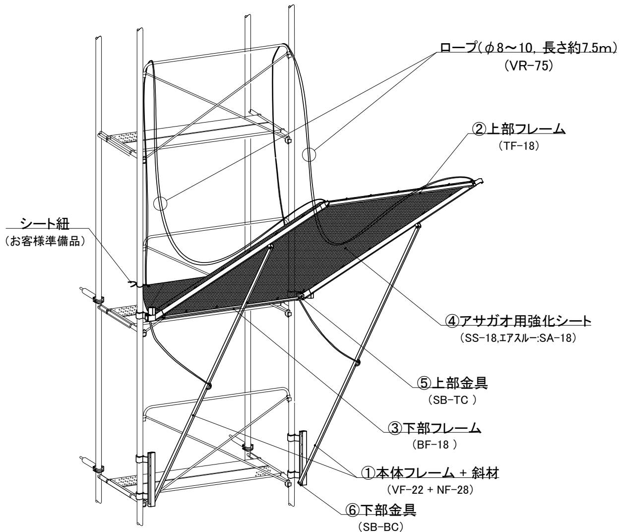
構成部材図（直線部）
